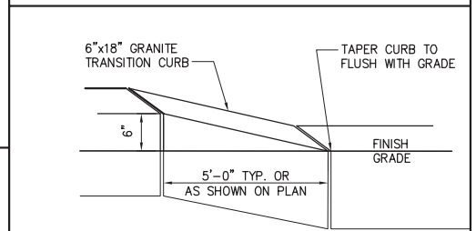
3 GRANITE CURB TERMINATION DETAIL SCALE: N.T.S.
